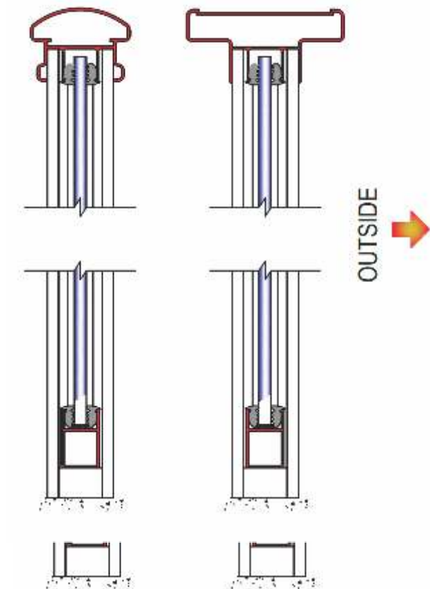
SECTION A-A
