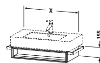
# VE 6013 ↔ 800 mm → Vero # 032985 # VE 6014 ↔ 1000 mm → Vero # 032910 # VE 6015 ↔ 1200 mm → Vero # 032912 ↗ 446 mm
