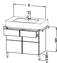
# VE 6413 ↔ 800 mm → Vero # 032985 # VE 6414 ↔ 1000 mm → Vero # 032910 # VE 6415 ↔ 1200 mm → Vero # 032912 ↗ 446 mm
