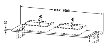
# VE 6271 L/R ↗ 311 mm
