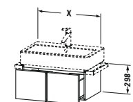
# VE 6103 ↔ 450 mm → Vero # 045450 # VE 6104 ↔ 550 mm → Vero # 045460 # VE 6105 ↔ 650 mm → Vero # 045470 # VE 6106 ↔ 750 mm → Vero # 045480 # VE 6107 ↔ 950 mm → Vero # 045410 # VE 6108 ↔ 1150 mm → Vero # 045412 ↗ 431 mm
