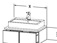
# VE 6550 ↔ 600 mm # VE 6551 ↔ 800 mm # VE 6552 ↔ 1000 mm ↗ 518 mm
