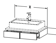
# VE 6560 ↔ 600 mm # VE 6561 ↔ 800 mm # VE 6562 ↔ 1000 mm ↗ 518 mm
