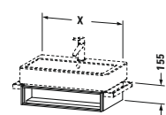
# VE 6003 ↔ 450 mm → Vero # 045450 # VE 6004 ↔ 550 mm → Vero # 045460 # VE 6005 ↔ 650 mm → Vero # 045470 # VE 6006 ↔ 750 mm → Vero # 045480 # VE 6007 ↔ 950 mm → Vero # 045410 # VE 6008 ↔ 1150 mm → Vero # 045412 ↗ 431 mm
