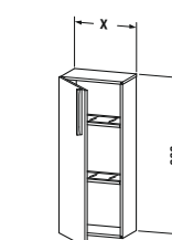
# VE 1105 ↔ 400 mm # VE 1155 ↔ 500 mm ↗ 240 mm
