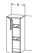
# VE 1106 ↔ 400 mm # VE 1156 ↔ 500 mm ↗ 360 mm
