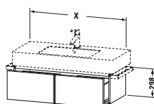
# VE 6113 ↔ 800 mm → Vero # 032985 # VE 6114 ↔ 1000 mm → Vero # 032910 # VE 6115 ↔ 1200 mm → Vero # 032912 ↗ 446 mm
