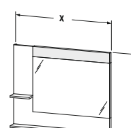
# VE 7310 ↔ 650 mm ⌀ 1 x 11 W # VE 7311 ↔ 800 mm ⌀ 1 x 14 W # VE 7312 ↔ 1000 mm ⌀ 1 x 18 W # VE 7313 ↔ 1200 mm ⌀ 1 x 22 W # VE 7314 ↔ 1400 mm ⌀ 1 x 28 W ↗ 142 mm IP 44 LED A++
