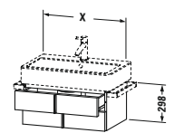
# VE 6203 ↔ 450 mm → Vero # 045450 # VE 6204 ↔ 550 mm → Vero # 045460 # VE 6205 ↔ 650 mm → Vero # 045470 # VE 6206 ↔ 750 mm → Vero # 045480 # VE 6207 ↔ 950 mm → Vero # 045410 # VE 6208 ↔ 1150 mm → Vero # 045412 ↗ 431 mm
