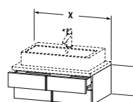
# VE 6570 ↔ 600 mm # VE 6571 ↔ 800 mm # VE 6572 ↔ 1000 mm ↗ 518 mm
