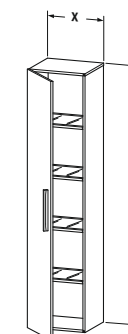
# VE 1116 ↔ 400 mm # VE 1166 ↔ 500 mm ↗ 360 mm
