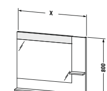
# VE 7320 ↔ 650 mm ⌀ 1 x 11 W # VE 7321 ↔ 800 mm ⌀ 1 x 14 W # VE 7322 ↔ 1000 mm ⌀ 1 x 18 W # VE 7323 ↔ 1200 mm ⌀ 1 x 22 W # VE 7324 ↔ 1400 mm ⌀ 1 x 28 W ↗ 142 mm IP 44 LED A++
