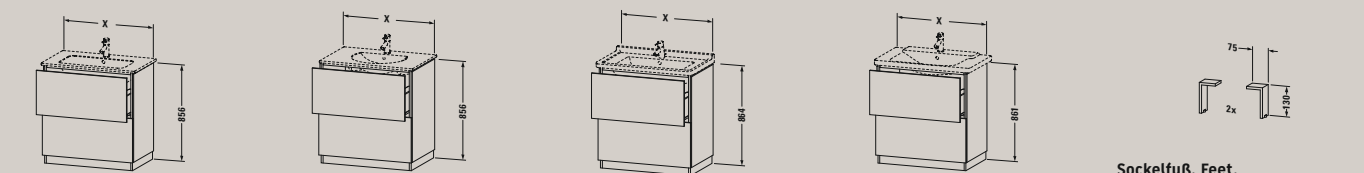
Sockelfuß. Feet. Patatas para mueble
