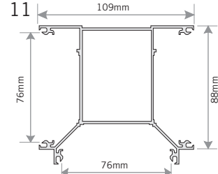
3 Way Box Post Die 6342 (FA 570)
