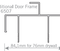
Traditional Door Frame Die 6508
