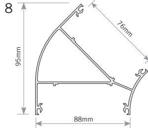
135° Corner Post Die 6324 (FA 550)
