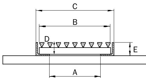
EZI-WALK Class A
